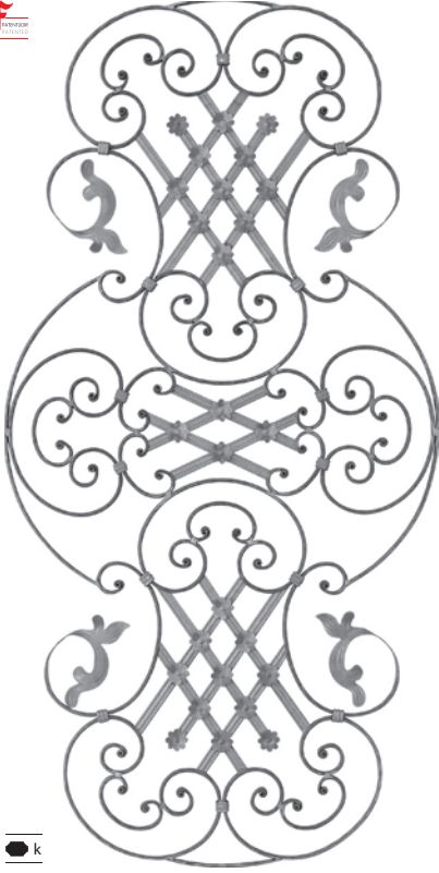
19731 80x160 cm. 19,600 kg. ■ 16x8 mm.
