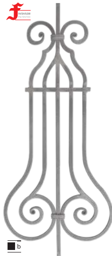
12676 35x80 cm. 5,128 kg. ■ 12 mm.
