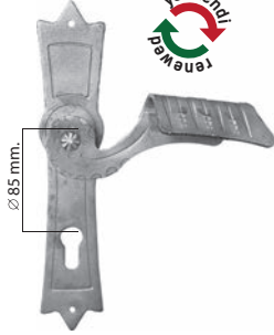
19786 B= 5,2 cm. H= 26 cm. 1,170 kg. Takım/Pair
