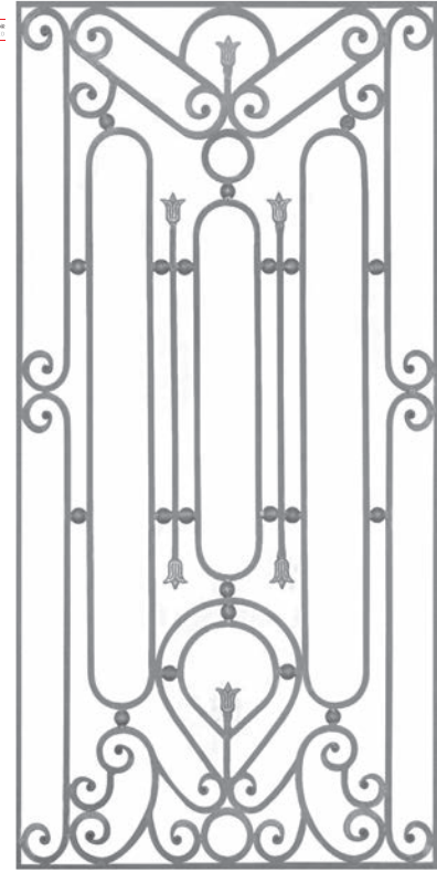
19741 80x160 cm. 30,480 kg. ■ 12 mm.
