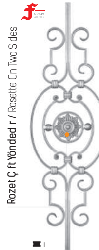
Rozet Ç ft Yönded r / Rosette On Two S des 168087 22x80 cm. 4,750 kg. — 16x8 mm.
