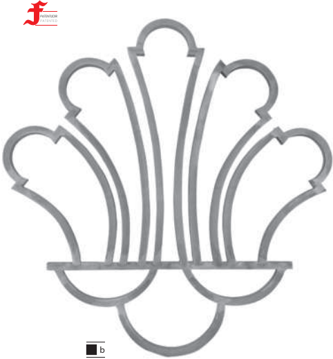
121243 53x55 cm. 5,120 kg. ■ 12 mm.
